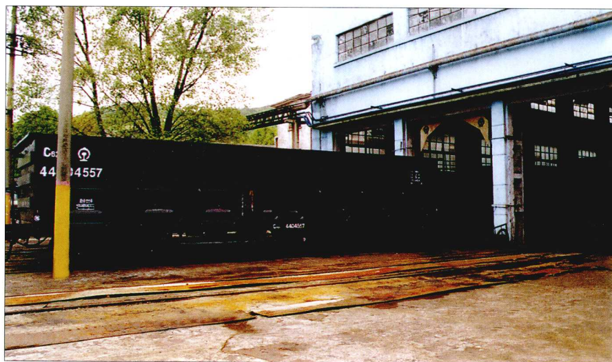
银行贷款支持的铁道部贵阳车辆厂即将出厂的新车箱
