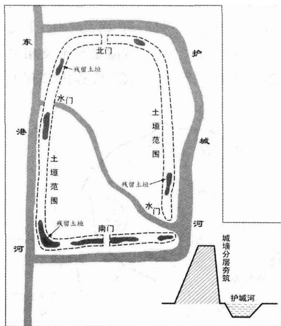
图2 湖北马家院出土的原始城堡 (据施元龙《中国筑城史》改绘)
