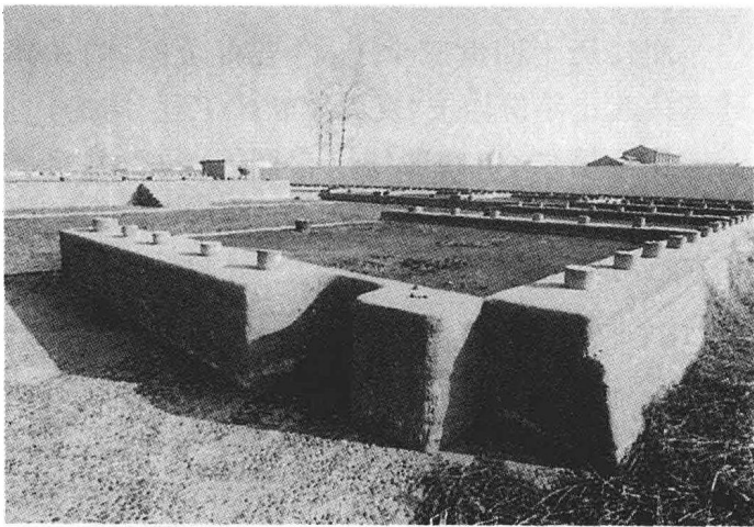
图5 偃师商城官殿区遗址现场
