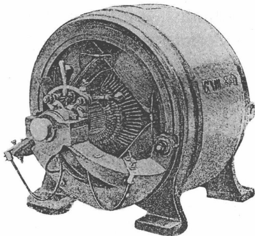
雅各布公司制造的电动机
