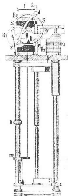
雅各布公司制造的弧光灯
