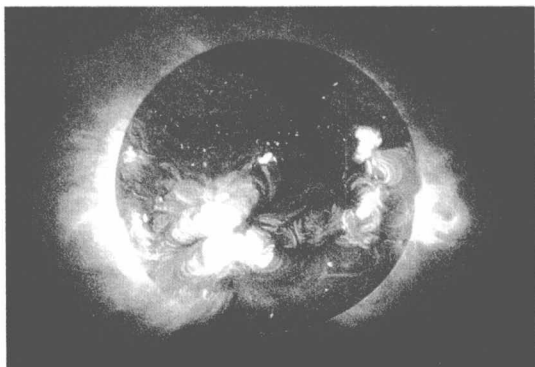
高倍太空望远镜下的太阳
