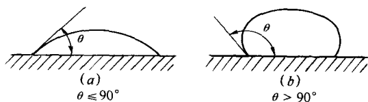
图 20-1 材料润湿示意图 (a) 亲水性材料; (b) 憎水性材料
