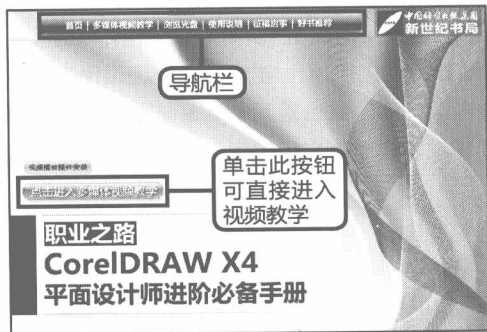
图1 光盘主界面
