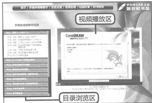
图2 播放界面
