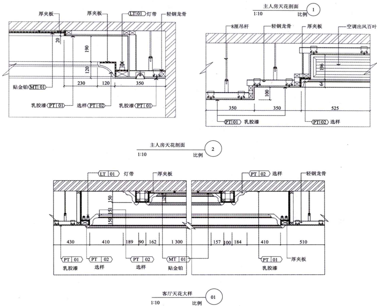
图 1-11 别墅设计剖面图和大样图 文健 石树勇 设计
