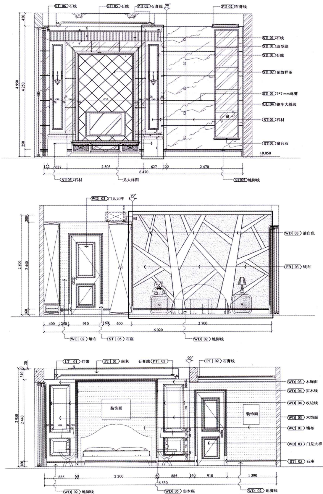
图 1-10 别墅设计立面图 文健 赵成余 设计
