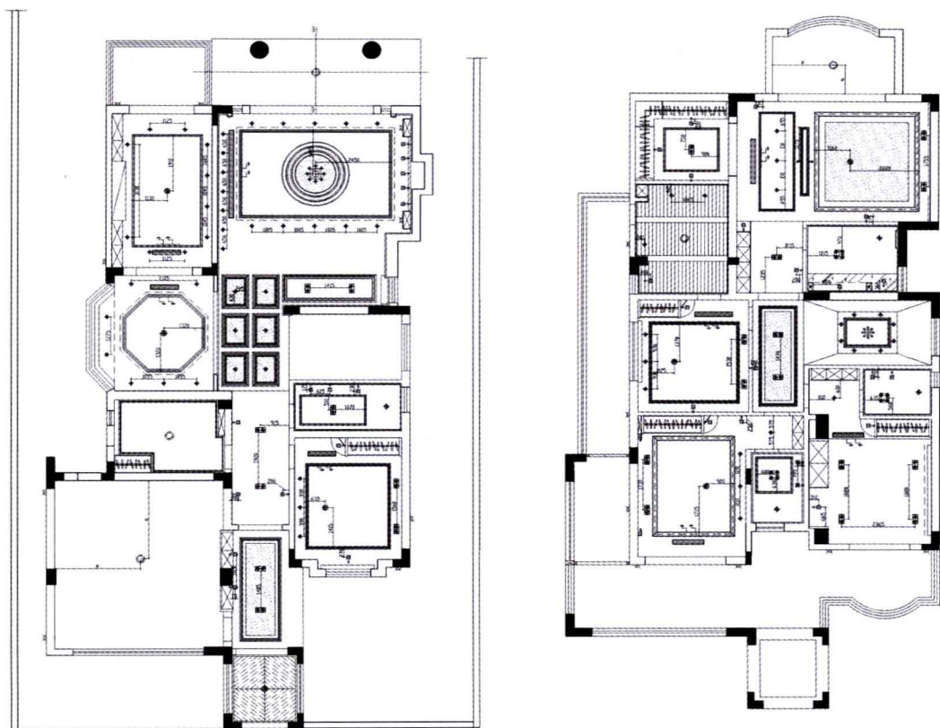
图 1-9 别墅设计天花图 文健 赵成余 设计
