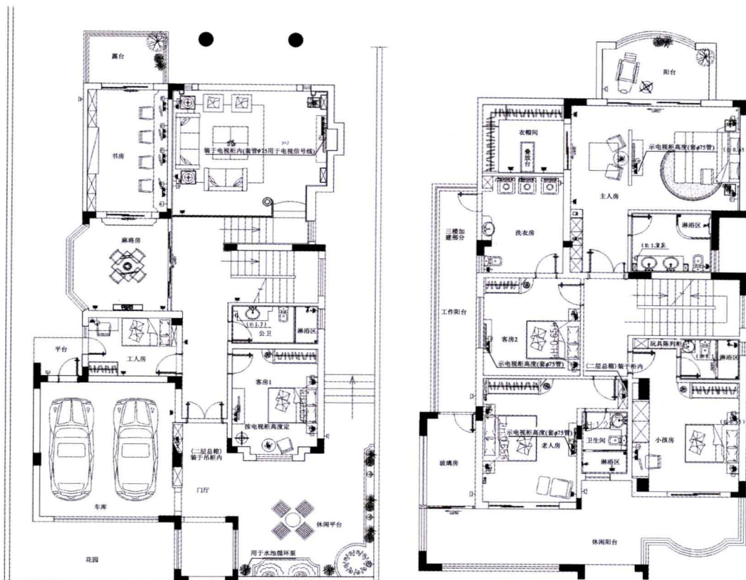
图 1-8 别墅设计平面图 文健 赵成余 设计
