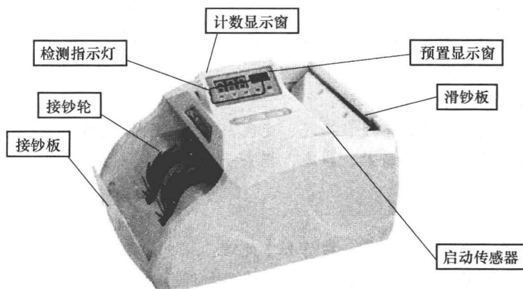
图 0.4 点钞机结构
