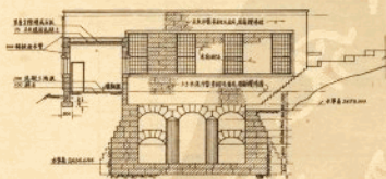
剖面丙
