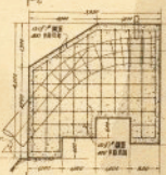
详图
