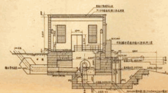
剖面乙
