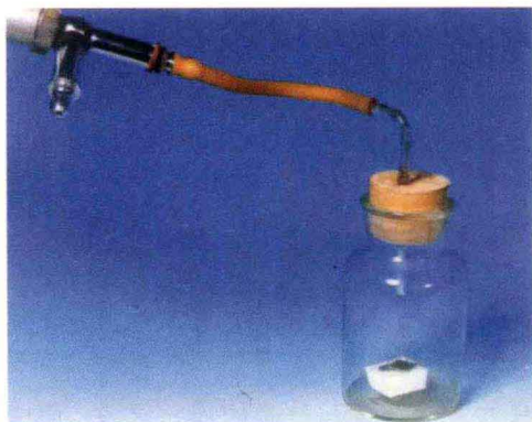
图1.2.7 真空不能传声
