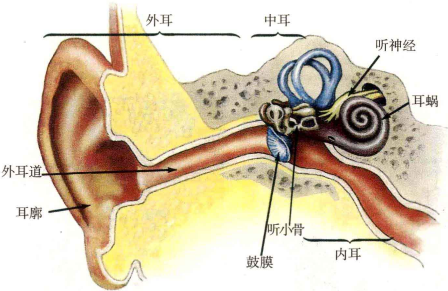
图 1.1.5 耳的结构示意图
