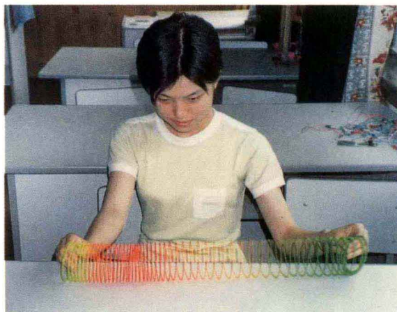
图1.2.8 塑料圈的振动
