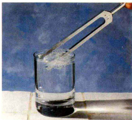
图1.2.1 音叉放入水中
