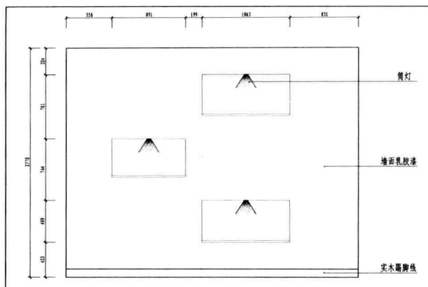
图 1-4 玄关南立面图
