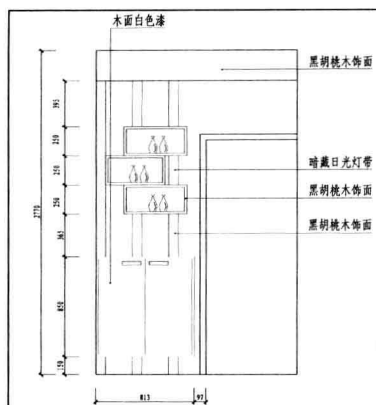
图 1-3 玄关北立面图
