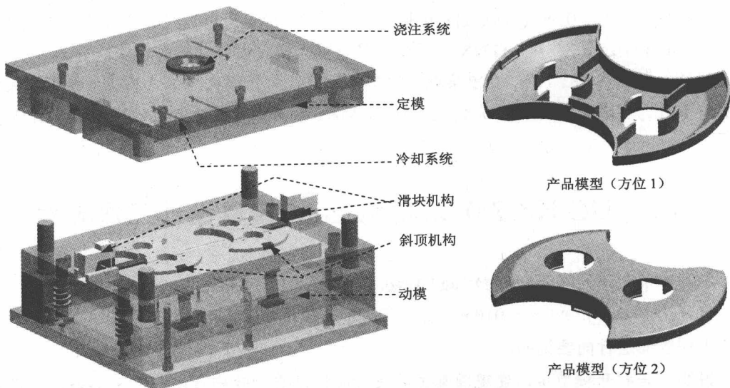
图 1.1.6 Mold Wizard 7.0 模架设计
