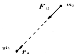
图 1-5 引力矢量
