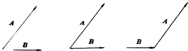
图 1-4 矢量平移
