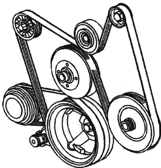
图 1-6-2 2003—2009 年款 ESCALADE 轿车传动皮带盘绕图
