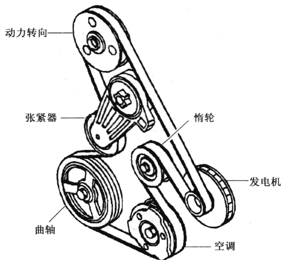
图 1-3-1 DEVILLE(4.6L 发动机)轿车传动皮带盘绕图
