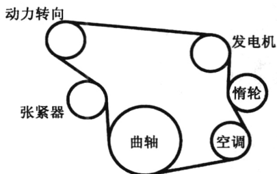
图 1-7-1 SEVILLE SLS 轿车传动皮带盘绕图
