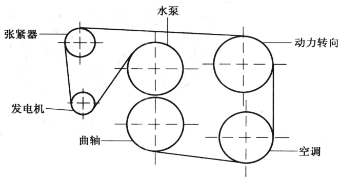
图 1-1-1 CATERA 轿车传动皮带盘绕图
