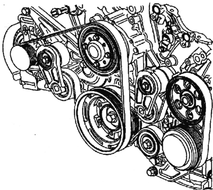
图 1-2-2 CTS(3.6L 发动机)轿车传动皮带盘绕图
