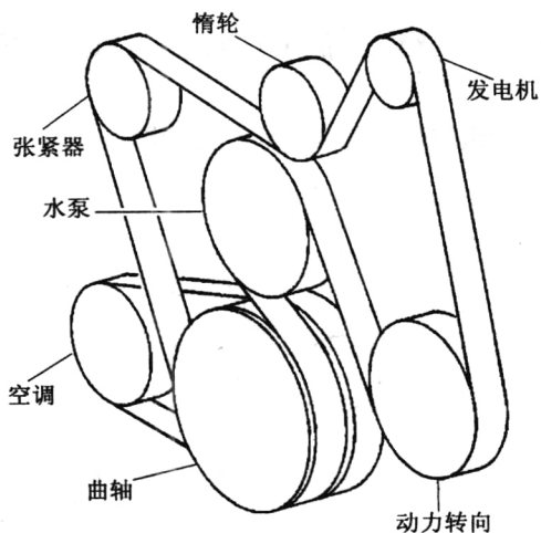
图 1-6-1 2000—2002 年款 ESCALADE 轿车传动皮带盘绕图
