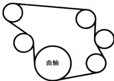
图 1-5-1 ELDORADO 轿车传动皮带盘绕图
