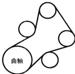
图 1-2-1 CTS(2.8L 发动机)轿车传动皮带盘绕图
