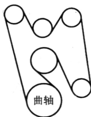
图 1-2-3 CTS(5.7L 和 6.0L 发动机)轿车传动皮带盘绕图
