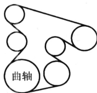
图 1-4-1 DTS(V8 4.6L 发动机)轿车传动皮带盘绕图
