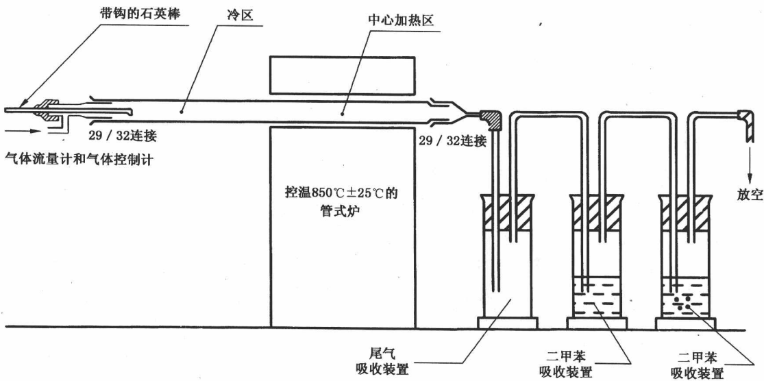
图 1 管式炉装置
