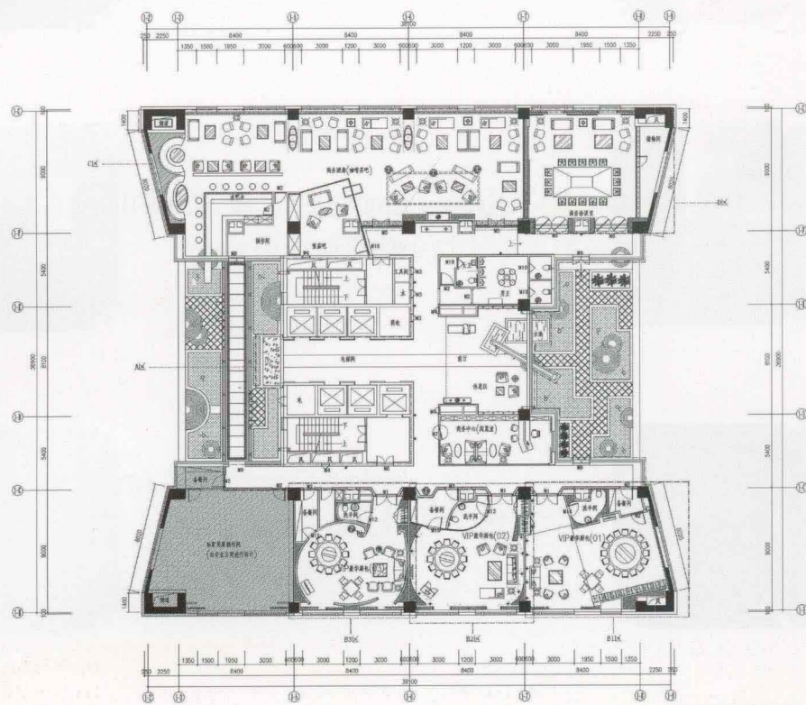
二十六层平面布置图
