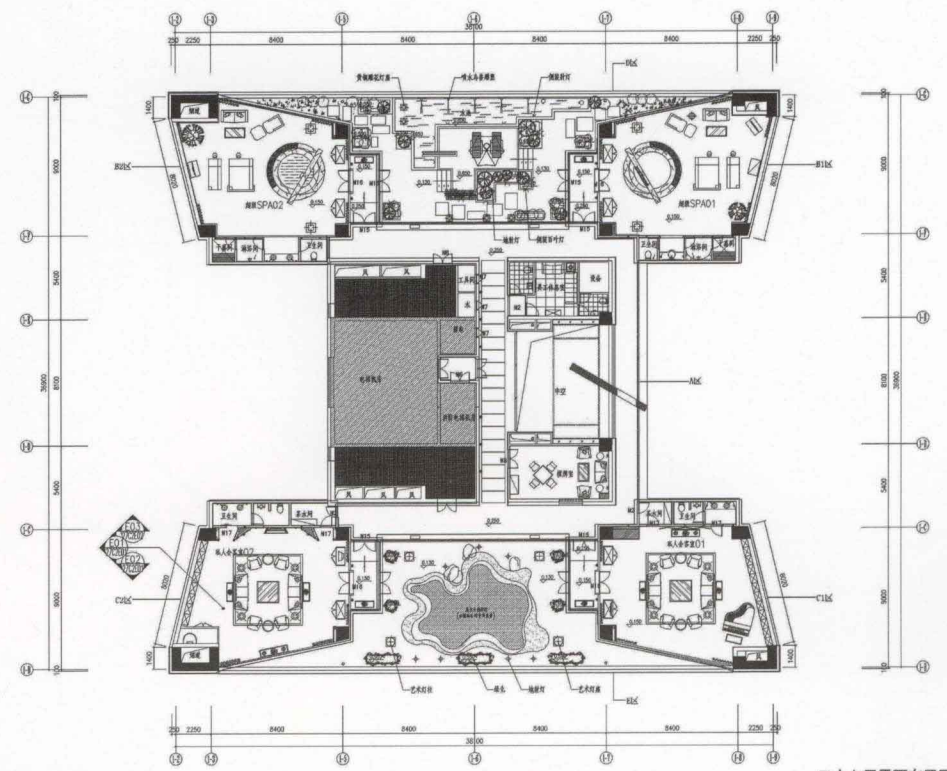
二十七层平面布置图
