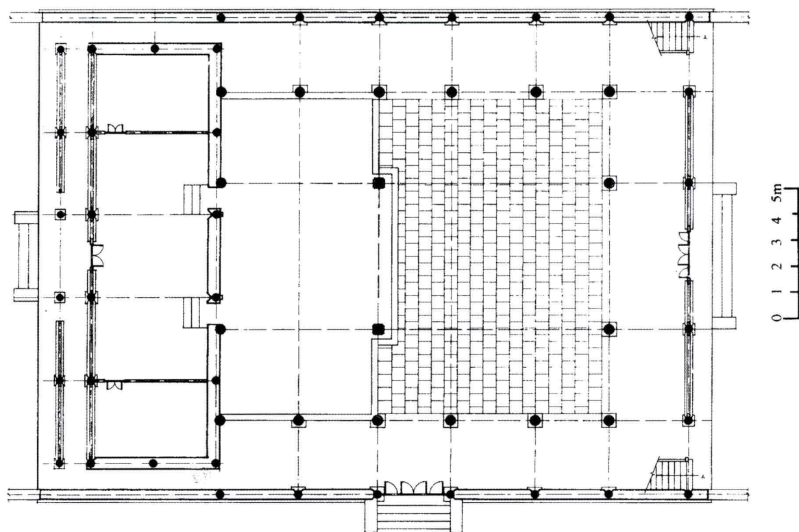
北京安徽会馆剧场平面 (取自《宣南鸿雪图志》 中国建筑工业出版社 1997年版)
