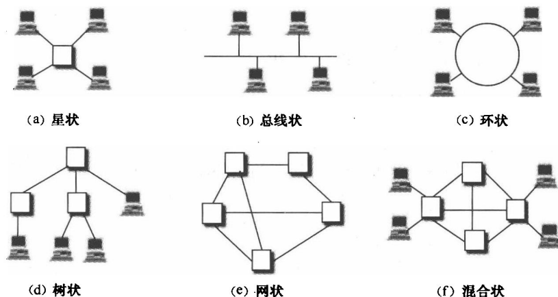
图 1.2 各种网络拓扑结构
