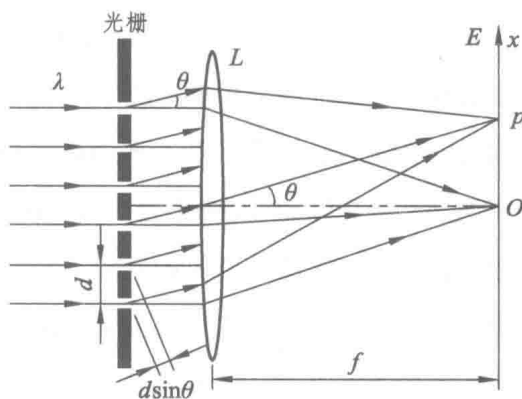
图 1.6 光栅衍射示意图
