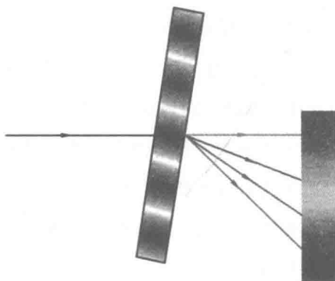
图 1.5 光栅衍射光谱示意图
