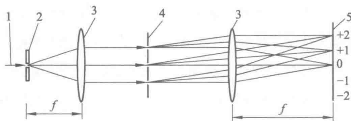
图 1.4 光栅衍射过程示意图
