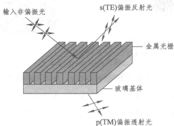
图 1.3 矩形金属偏振光栅结构图
