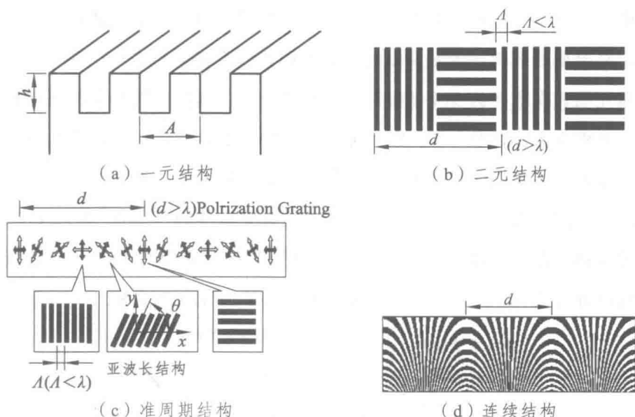
图 1.2 不同光栅周期结构示意图
