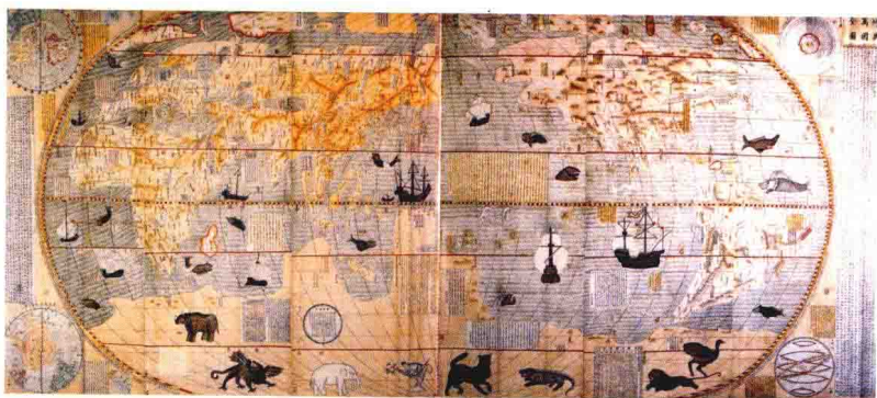
图9 明 坤輿万国全图
