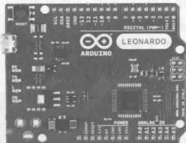
图 1-5 Arduino Leonardo
