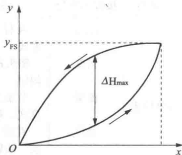
图 1-1 仪表变差特性图
