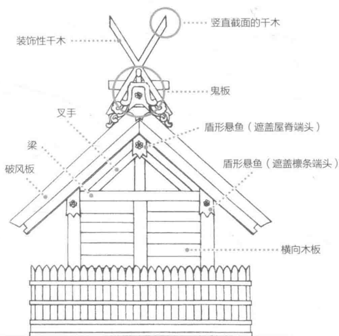
本殿背立面图
