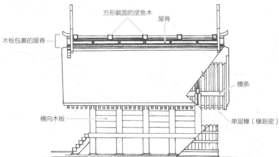
本殿侧面图
