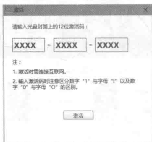
图1“激活”对话框
