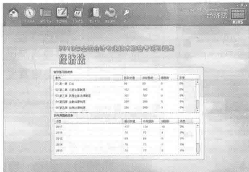
图2“首页”板块
