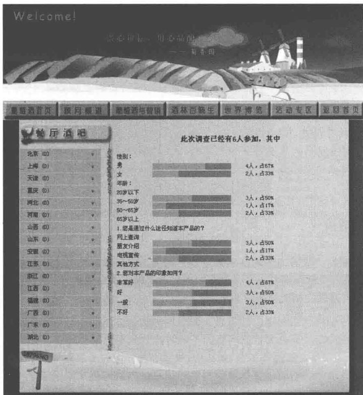
图 1-2 动态网页
