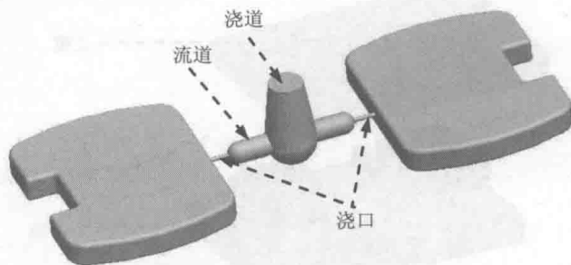
图 1.1.4 浇注系统
