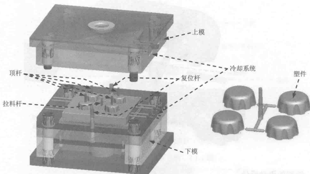
图 1.1.7 EMX10.0 模架设计
