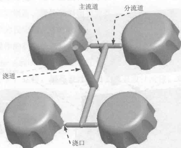
图 1.1.5 浇注系统 (含分流道)
