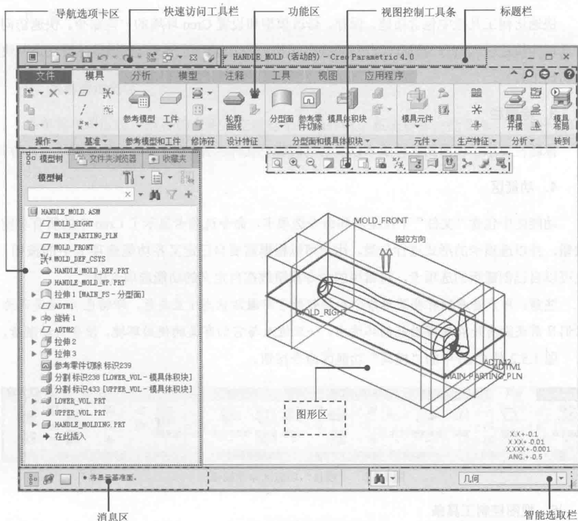
图 1.5.1 Creo 4.0 模具工作界面
