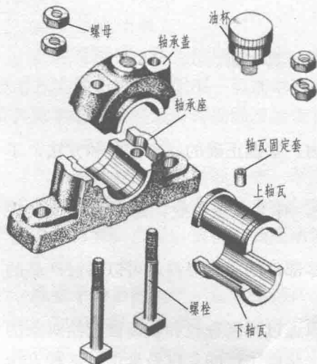
图 1-1 滑动轴承
