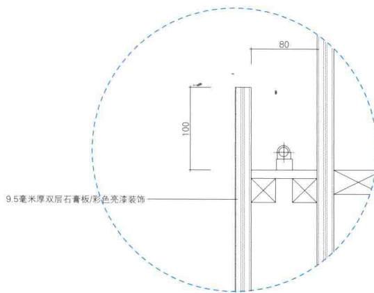
细节图D
