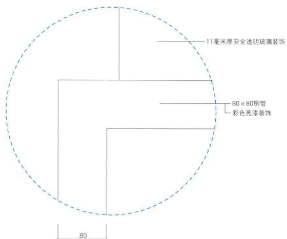
细节图F
