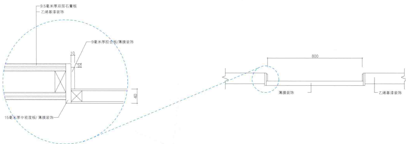
剖面图C
