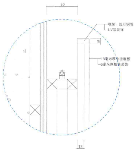
细节图E
