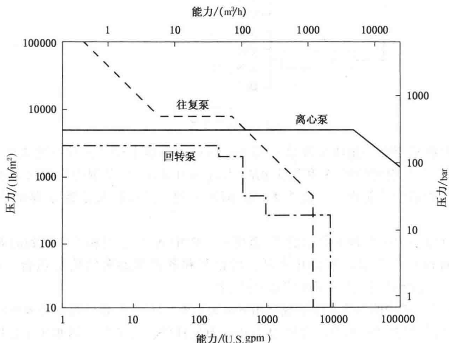
图 4 按分类, 泵压力与能力的近似上限
