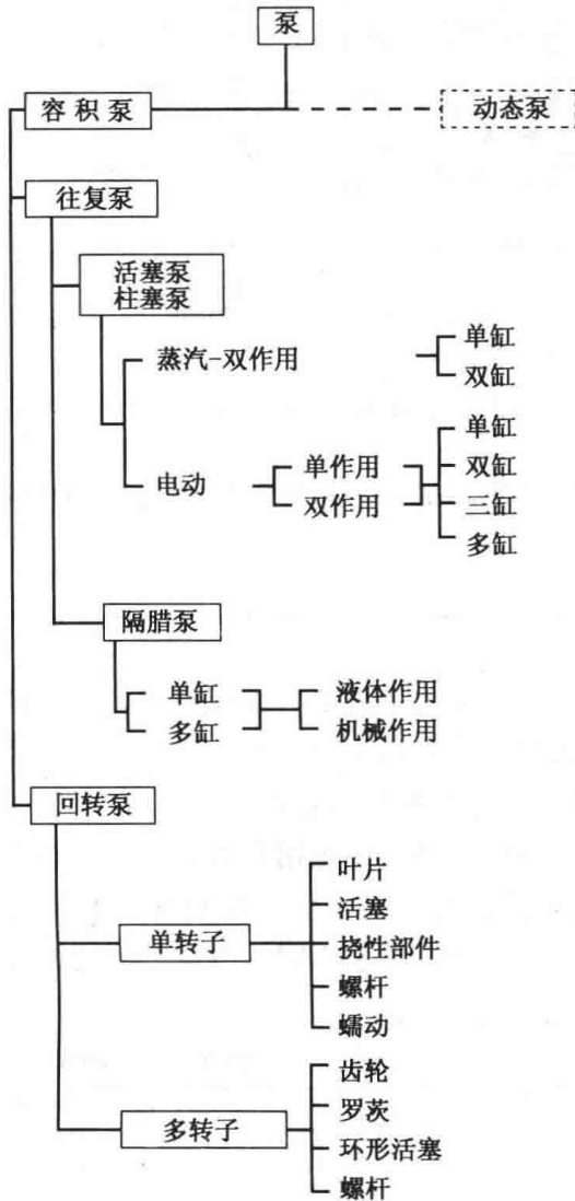
图 2 容积泵分类
