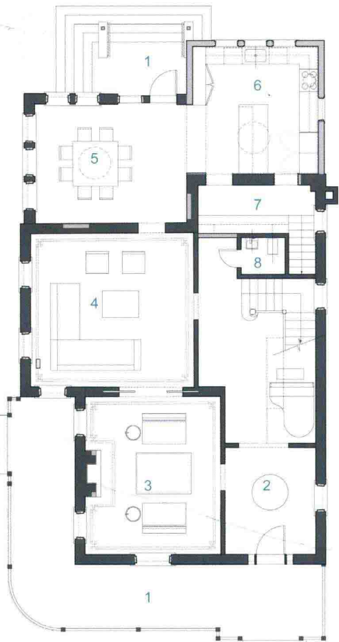
First Floor Plan 一层平面图
