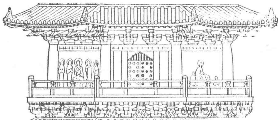
杭县闸口龙山白塔第一层立面
