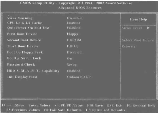
图 1.31 BIOS 特性设置
