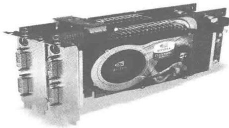
图 1.8 SLI 双显卡
