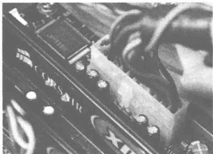
图 1.25 主板 ATX 电源的连接
