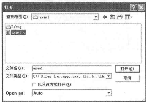
图 1-13 “打开”对话框
