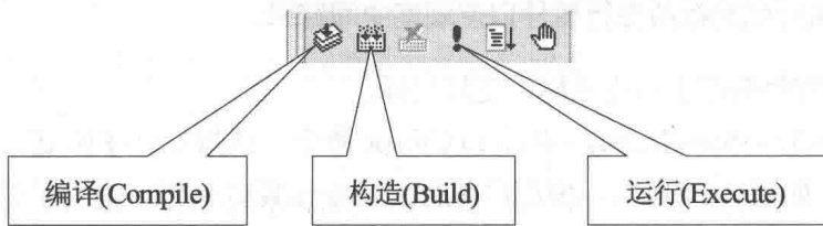
图 1-12 编译微型条
