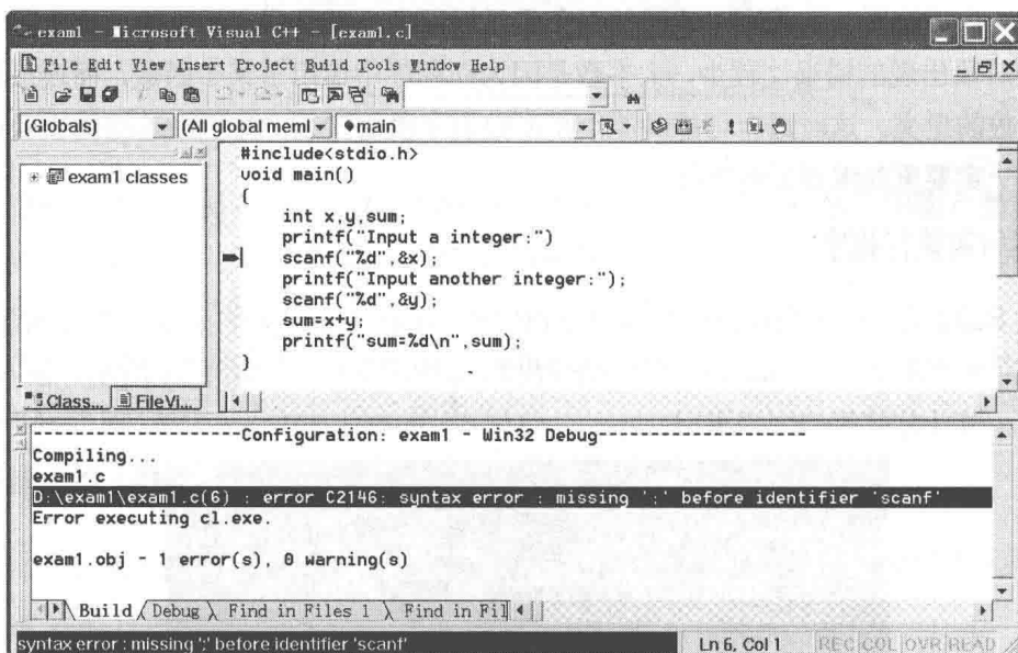
图 1-9 编译出错
