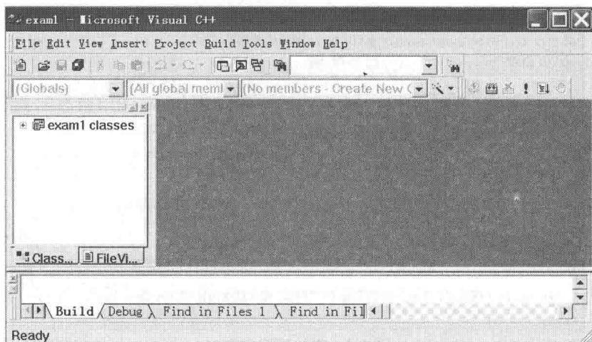
图 1-4 空项目窗口
