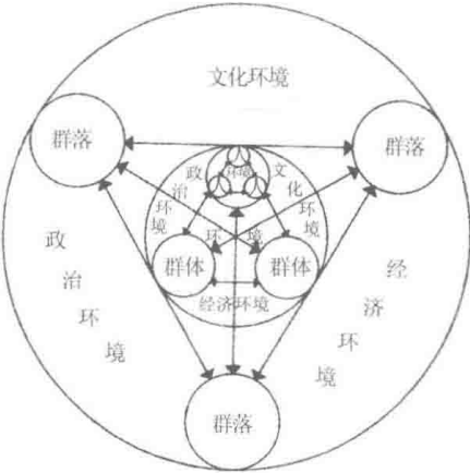
图 1-1 人文生态系统结构
