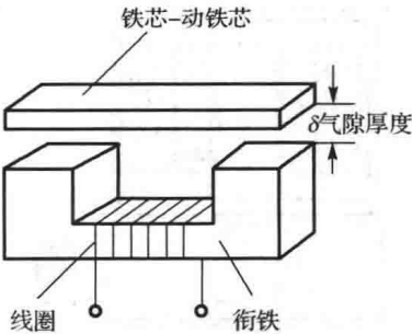
图 2-9 变气隙式电感传感器结构示意图
