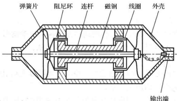
图 2-7 惯性式电动传感器结构示意图 [2]
