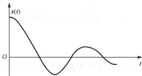
图 2-3 欠阻尼振动衰减曲线
