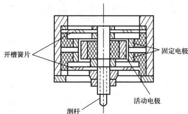
图 2-10 电容式传感器结构示意图 [2]
