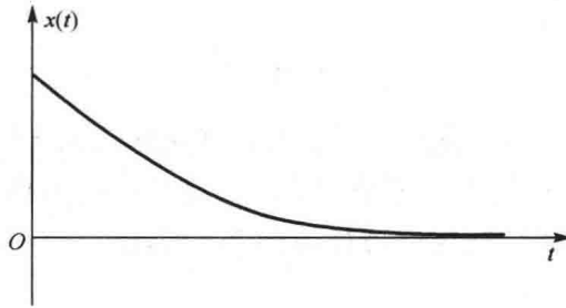
图 2-5 临界阻尼振动衰减曲线
