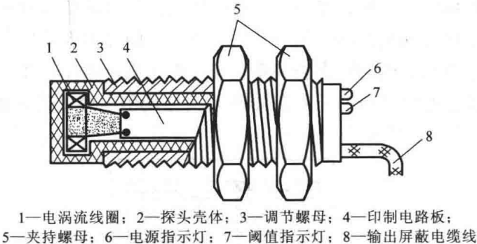
图 2-8 电涡流式位移传感器结构示意图
