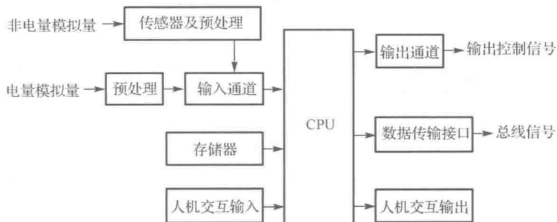
图 1.1 电子作品组成框图
