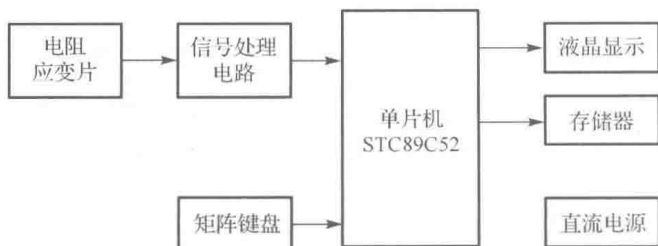
图 1.2 简易电子秤组成框图
