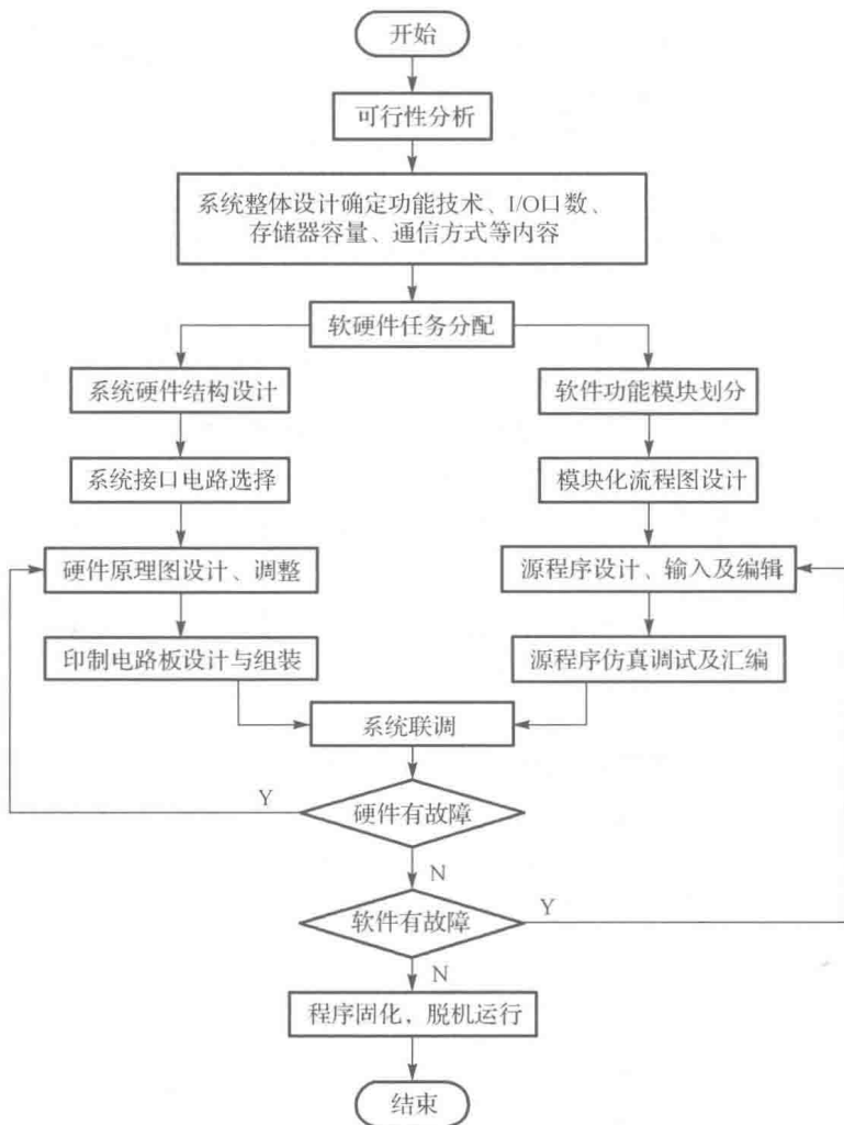
图 1.3 电子系统的开发流程
