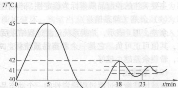
图 1-6 发酵过程控制系统的过渡过程响应曲线
