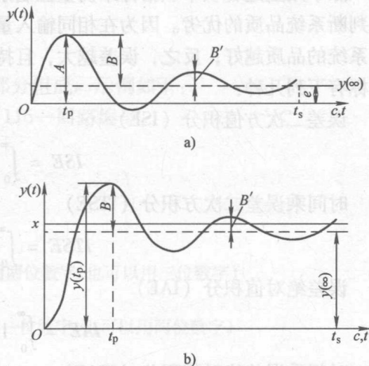
图1-5 阶跃作用下控制系统过渡过程响应曲线
