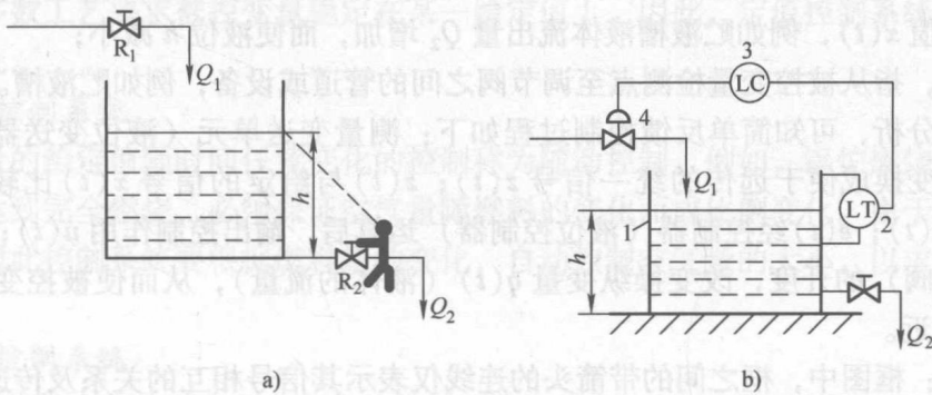
图 1-1 人工液位控制和自动液位控制
