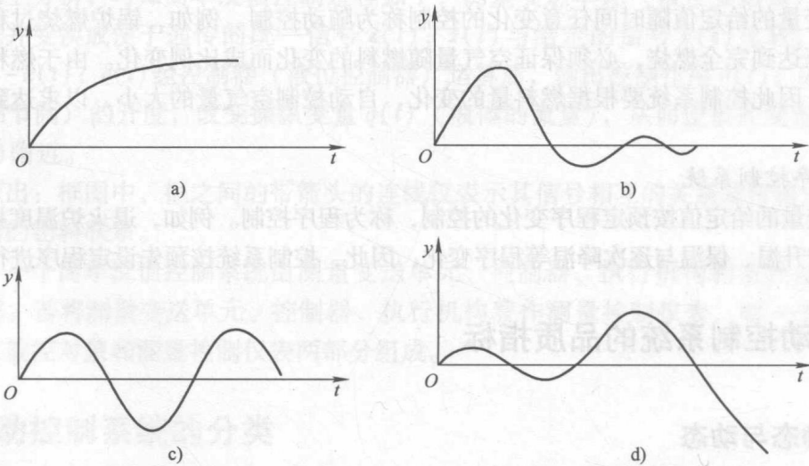
图 1-4 自动控制系统在阶跃输入作用下过渡过程的四种形式
