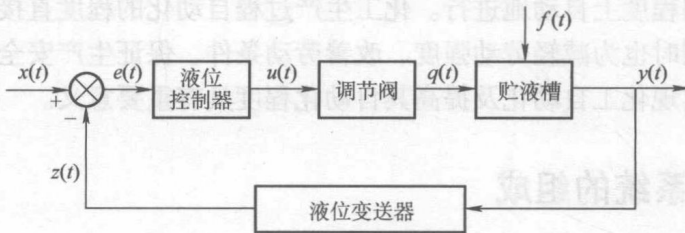
图 1-2 自动液位控制系统组成框图
