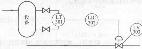
图 1-10 液位控制系统工艺管道及控制流程图示例
