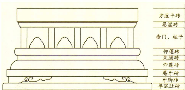
宋式须弥座各部位名称
