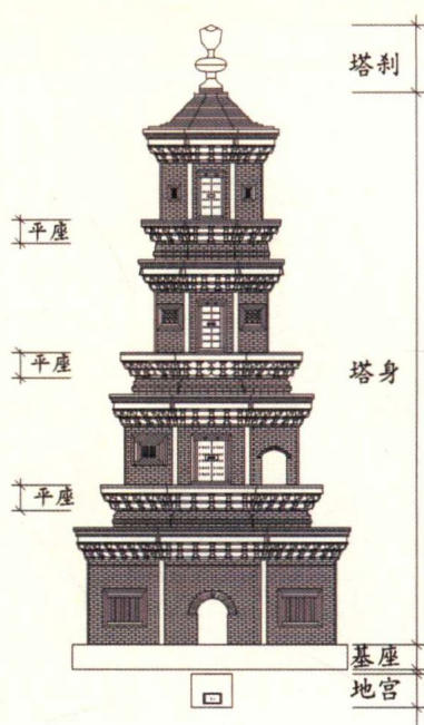
古塔结构组成图（一）
