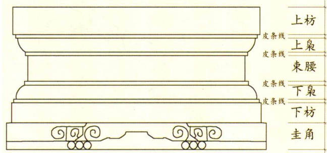
清式须弥座各部位名称
