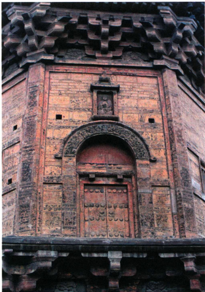
圆觉寺塔一层拱券门及斗拱细部
