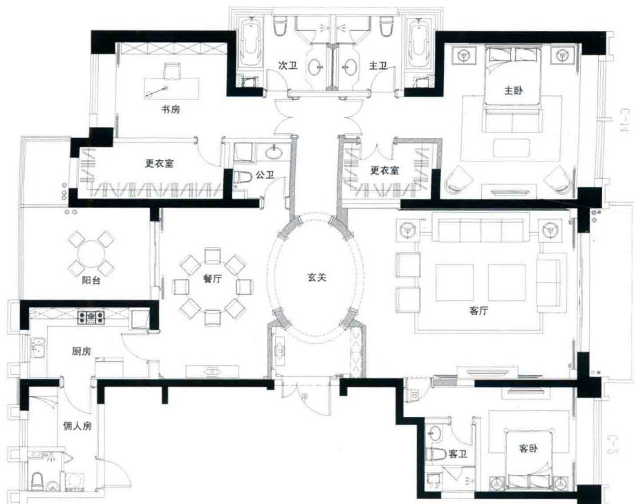
平面布置图
