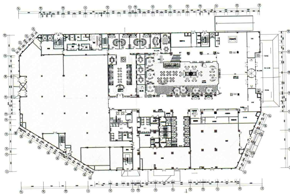
一层平面布置图
