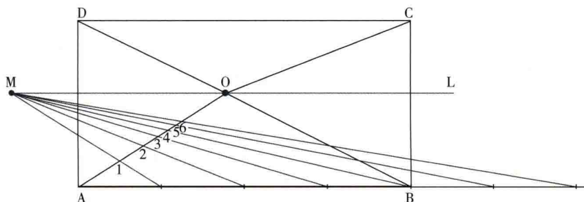
图2-4 步骤四图示
