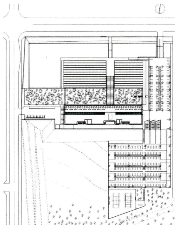
配置图 S=1/5000
