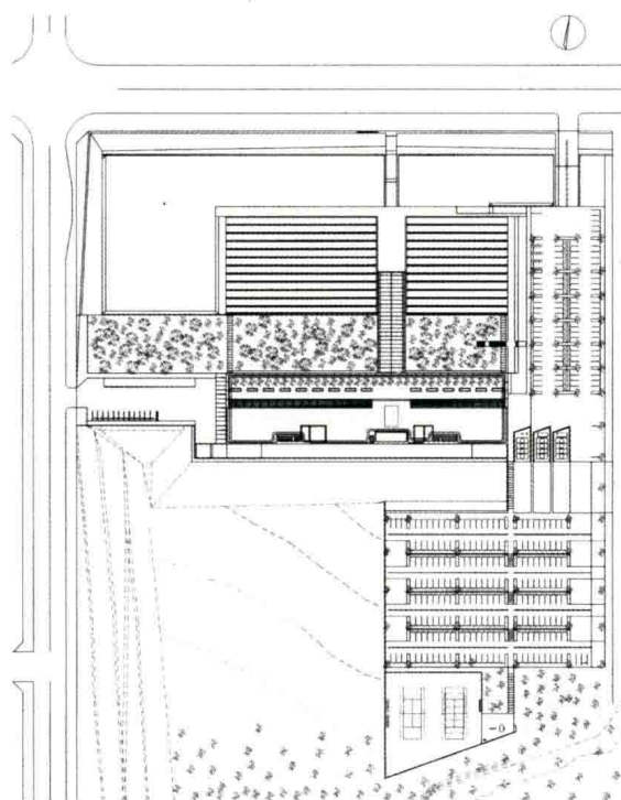
配置图 S=1/5000
