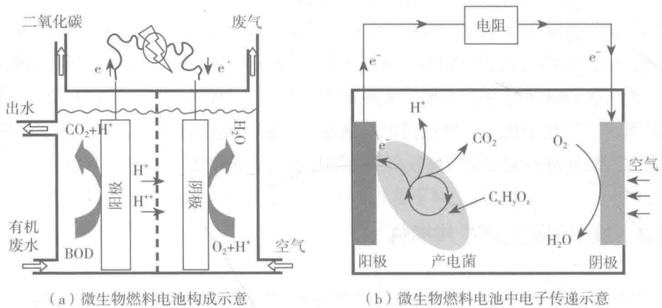
图1-2 微生物燃料电池示意
