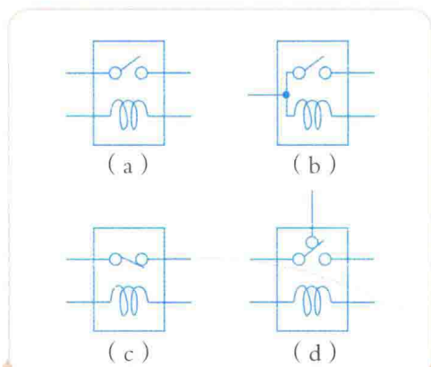
图 1-9 继电器按断开及接通方式分类
