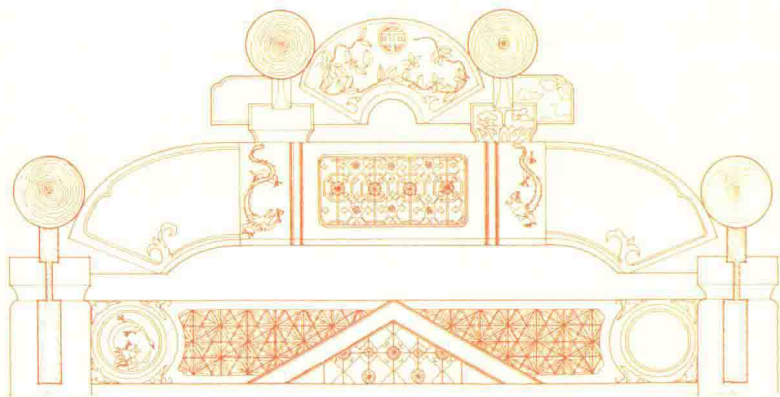
图1-4 江苏常熟彩衣堂包袱彩画二(章忠民 测绘)
