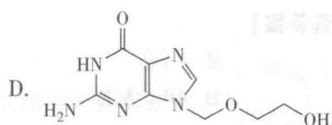
阿昔洛韦
