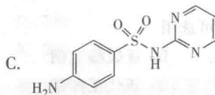
磺胺嘧啶
