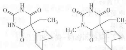
环己巴比妥
