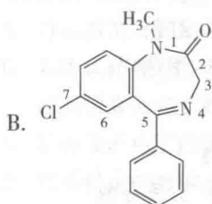
地西泮
