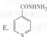
异烟肼
