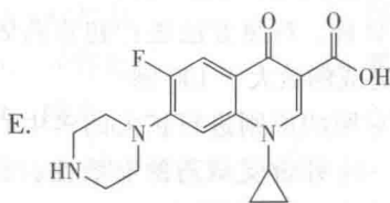
环丙沙星
