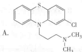
氯丙嗪
