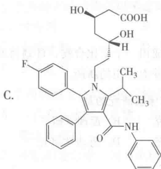
阿托伐他汀
