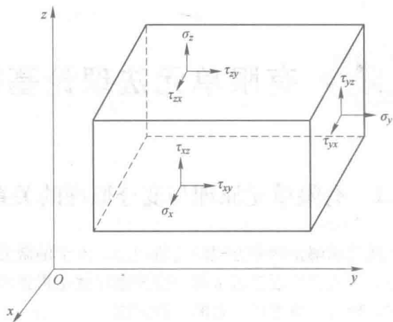
图 2-1 应力分量
