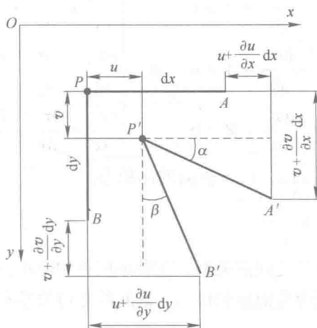
图 2-2 应变分量
