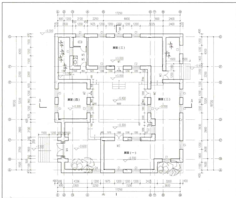
山东乡情展馆·平面尺寸图
