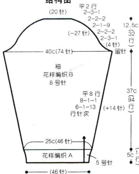
结构图
