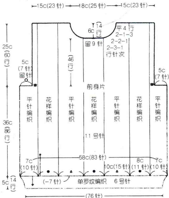
结构图
