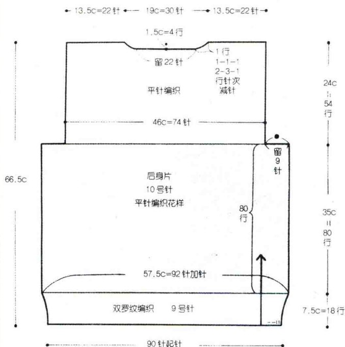
结构图
