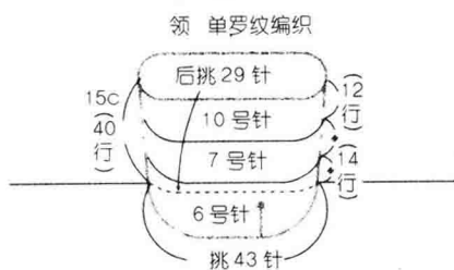
结构图
