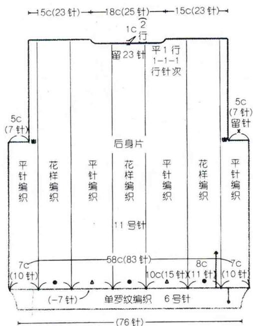
结构图
