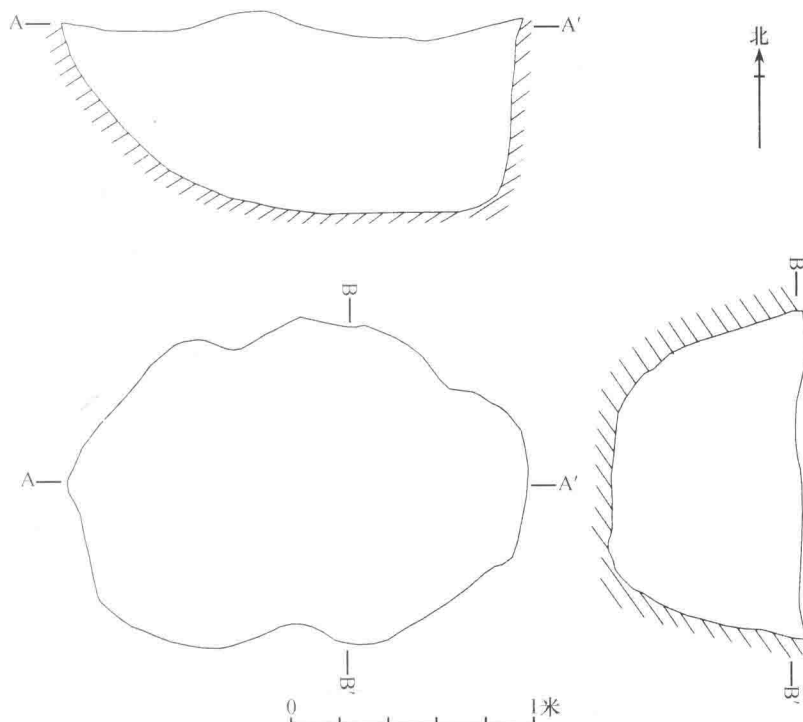
图六 H8平、剖面图
