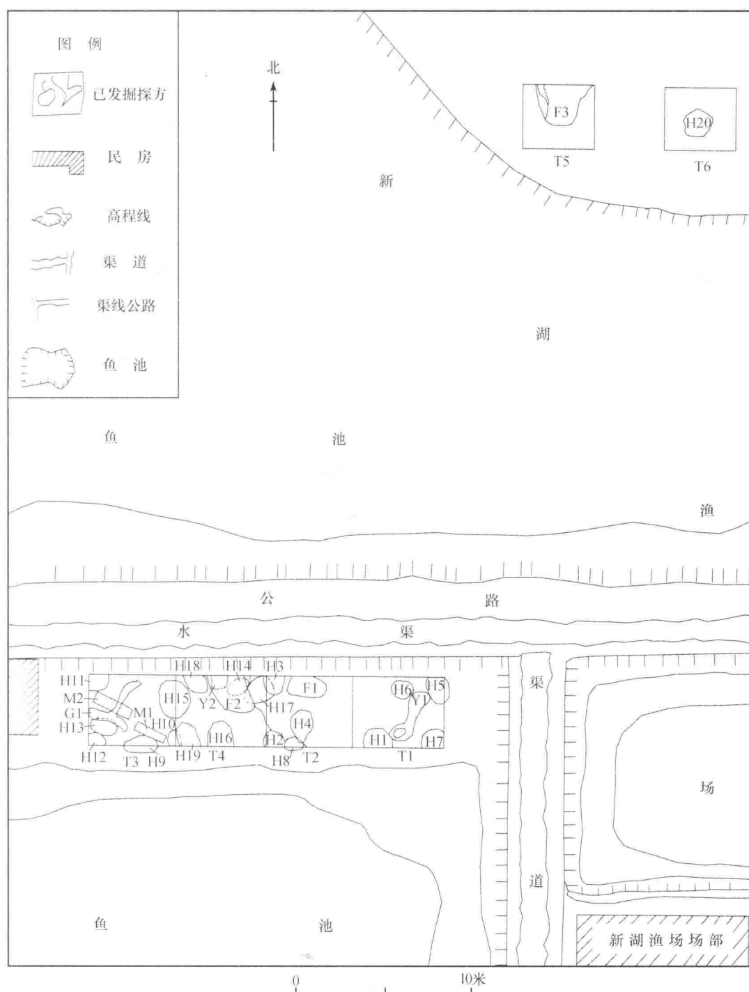
图二 新湖遗址探方、遗迹分布示意图
