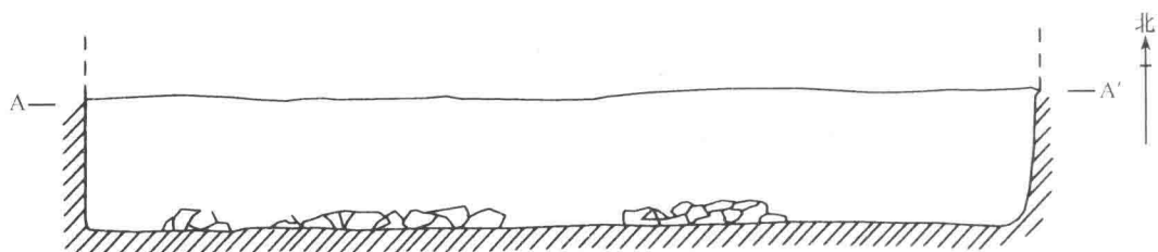
图七 M1平、剖面图
